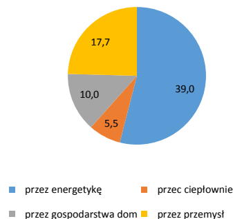
Zużycie węgla kamiennego* w 2018 roku [MT]
