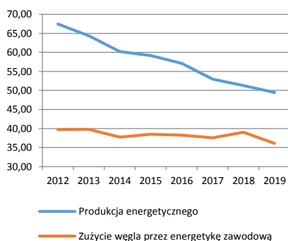
Produkcja i zużycie węgla* przez energetykę [MT]
